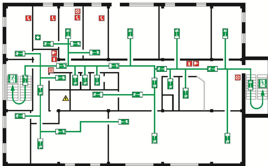
План 1 этажа
