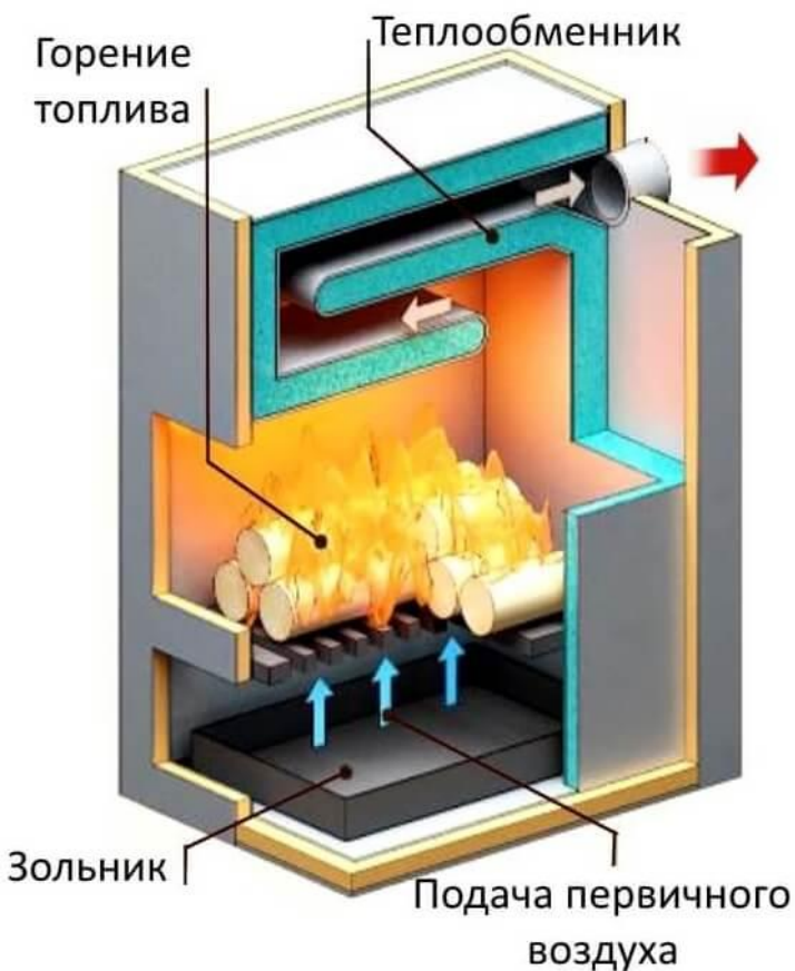
Обычный твердотопливный котел
