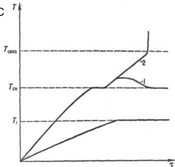
ПАРАМЕТРЫ УРАВНЕНИЙ, ХАРАКТЕРИЗУЮЩИХ САМОВОЗГОРАНИЕ
